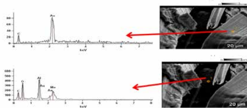
Figura 18 – EDS do PEAD puro e da inclusão de \text{Al}_2\text{Mo}_3\text{O}_{12} no nanocompósito com 1% de nanocarga
