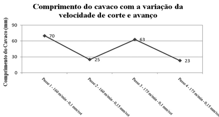
Figura 5. Variação do comprimento do cavaco em função da velocidade de corte e avanço
