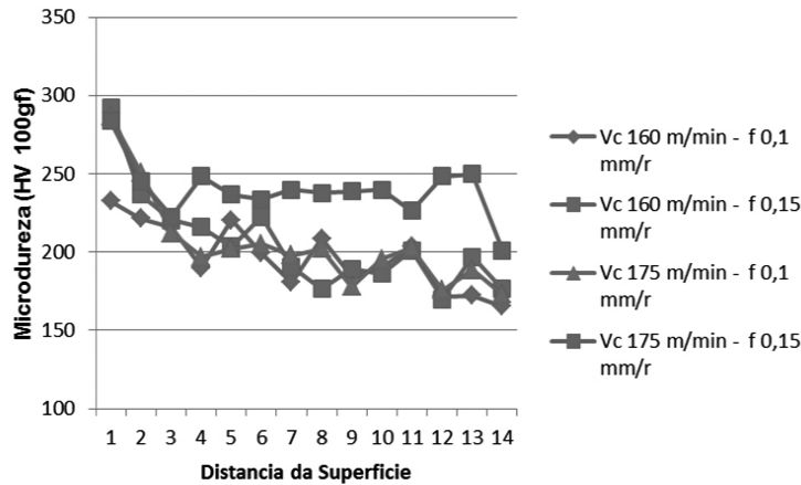
Figura 7. Microdureza média medida da próxima a extremidade ao centro a cada parâmetro de usinagem
