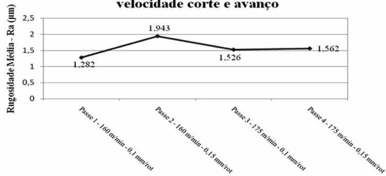
Figura 6. Variação da rugosidade média em função da velocidade de corte e avanço
