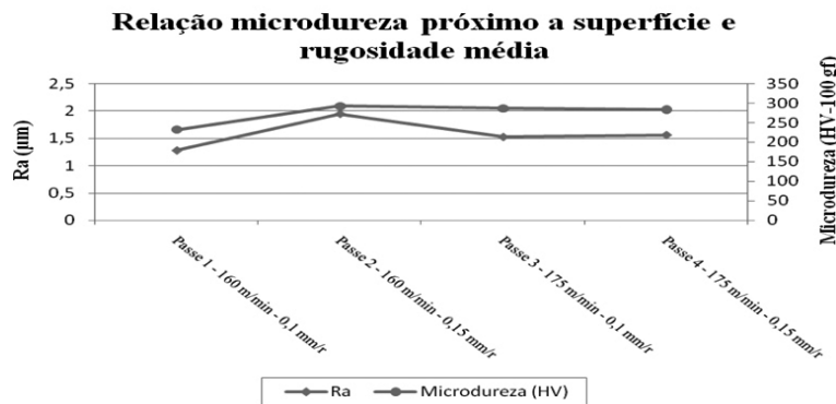
Figura 8. Comparação da rugosidade e microdureza média medida próxima à superfície até o centro
