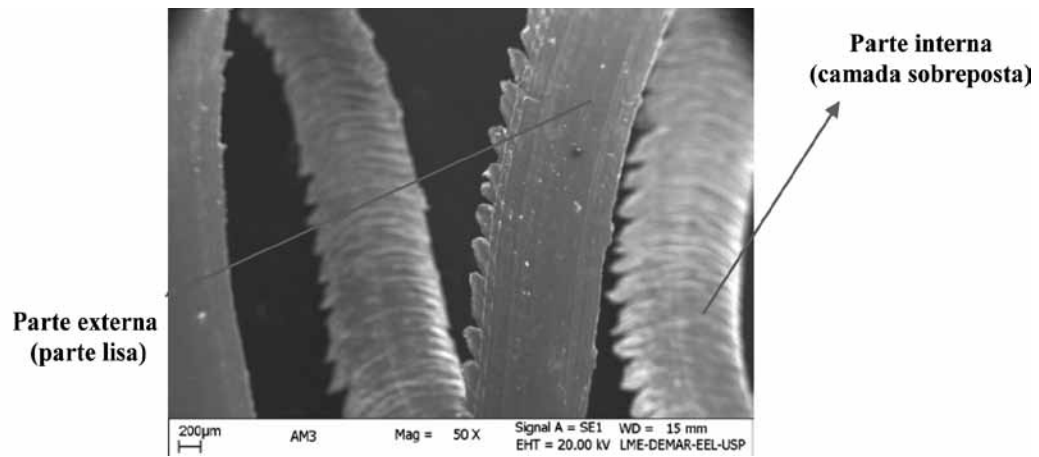
Figura 3. Morfologia do Cavaco ( V_c = 175 m/min e f = 0,1 mm/r)
