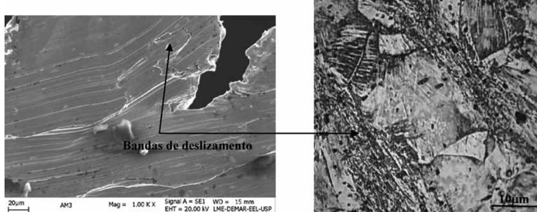
(a) Detalhe das bandas de deslizamento entre as zonas de recalque por meio de Microscopia Eletrônica de Varredura e (b) Detalhe das bandas de deslizamento por meio da Microscopia Óptica.
