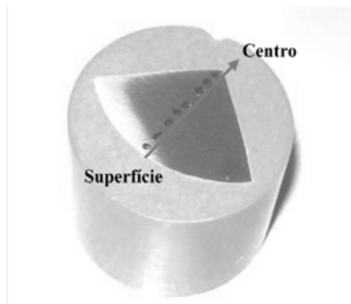
Figura 1. Corpo de Prova embutido e Sentido de medidas da microdureza
